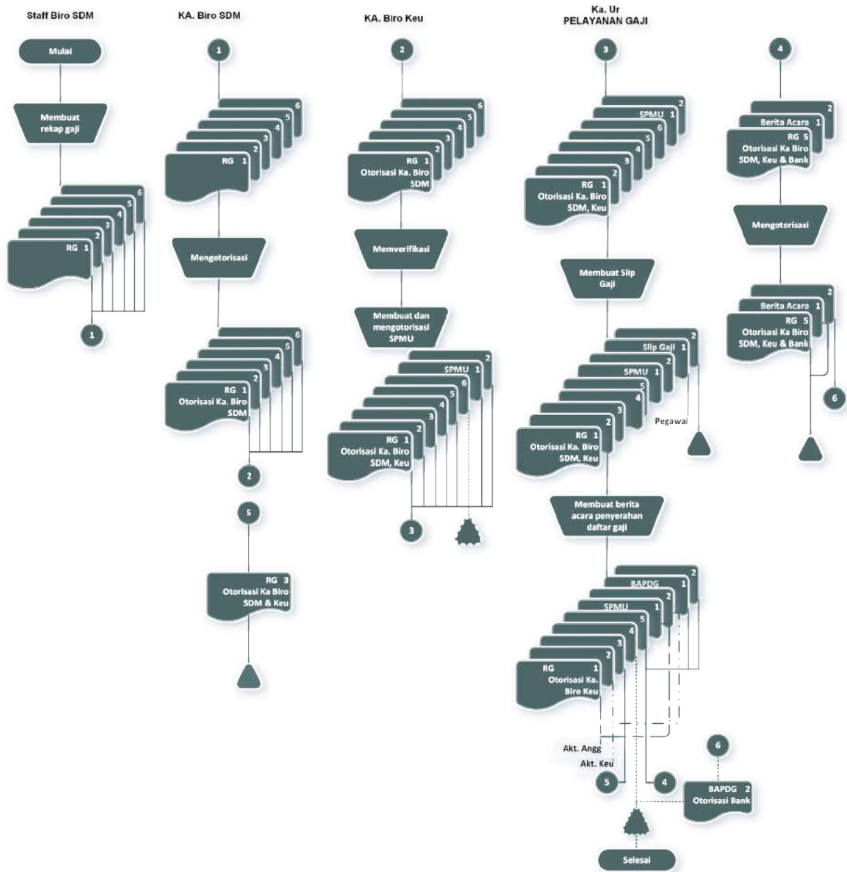
Flow chart Sistem Penggajian Dosen dan Karyawan (Manual)
